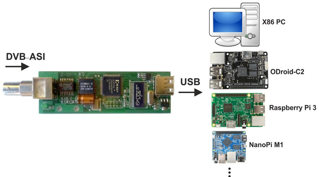
AUSB-2 : a DVB-ASI USB Card
